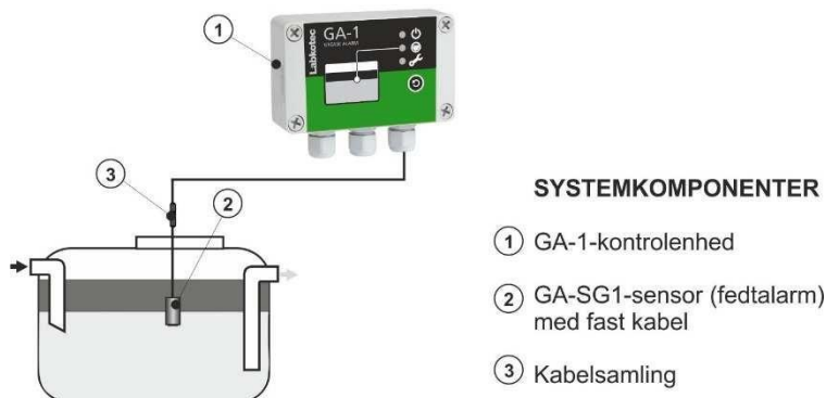
Figur 1. Overvågning af fedtudskiller med GA-1-alarmenhed
